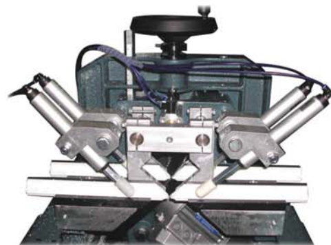
Simulatore 225 con 4 morse Sim 225 mit 4 Spannvorrichtungen
